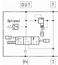
Schema di funzionamento Functional diagram
